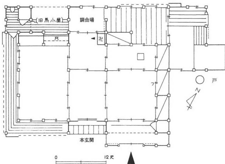
旧石井家平面図
