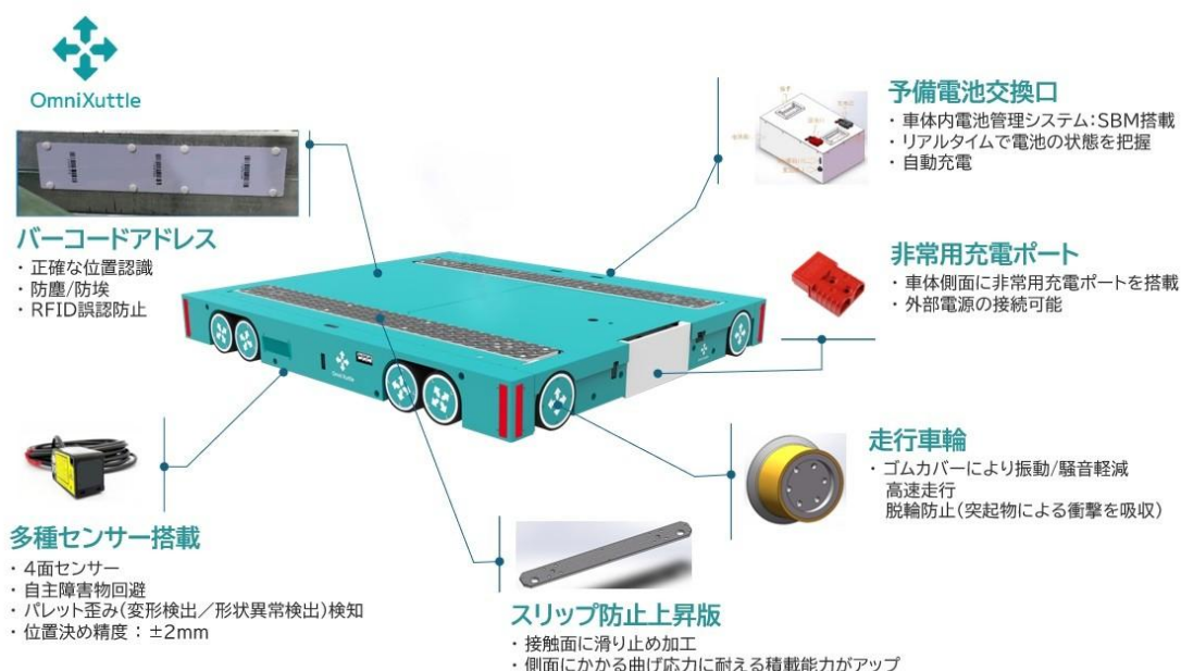
4 方向パレットシャトル
