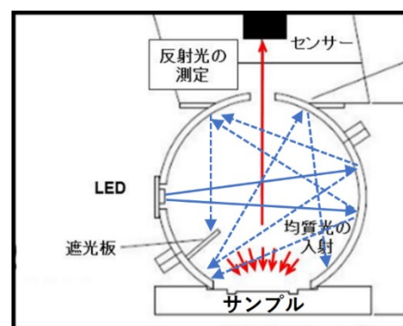
「CA-200」計測原理
