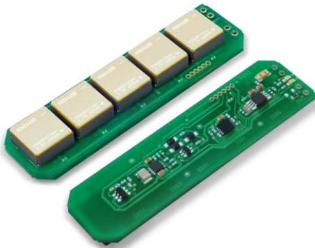
全固体電池電源モジュール 「SBM-DEMOBOARD-011」
