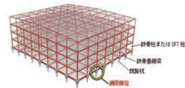
奥村式鉄骨基礎梁工法の適用部位
