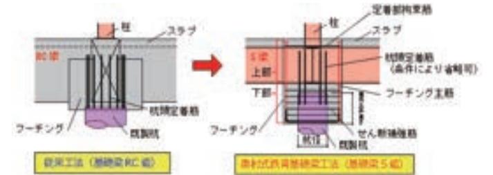
奥村式鉄骨基礎梁工法の概要
