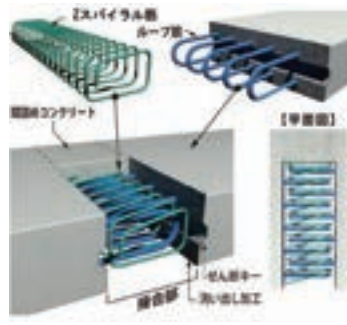
Zスパイラル工法の概要
