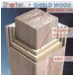
SHIELD WOOD®の構成
