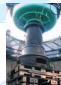
灯台レンズ用免震装置
