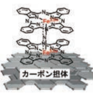
超強力酸化触媒の構造
