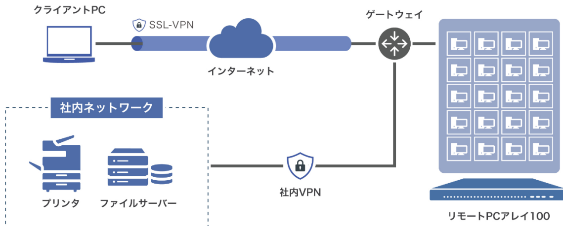
「at+link リモート PC サービス」システム概念図
