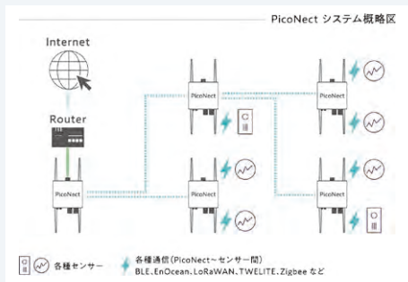
PicoNect概略図
