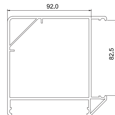
P6059 90° 拼接材
