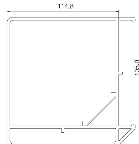
P8059 90° 拼接材
