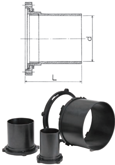
組合式穿樑接頭 Assembly type Beam Fittings 單位：mm
