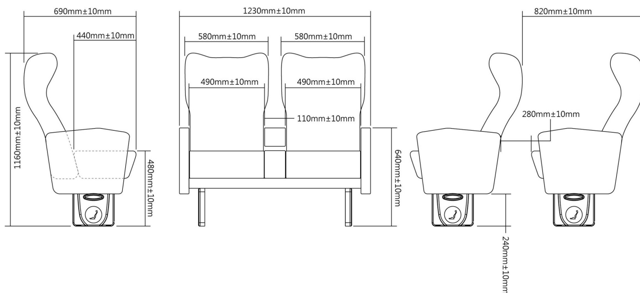
2D 規格圖
