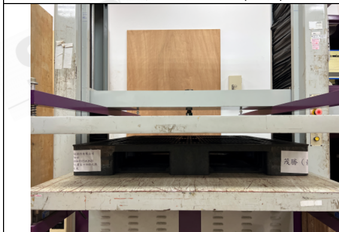
照片“E” 平面抗壓測試
