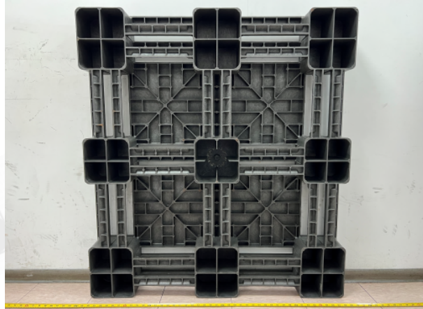
照片“B”樣品外觀：反面
