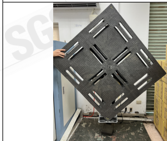
照片“C”墜落測試
