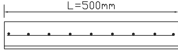
蓋板正面及鋼筋透視圖
