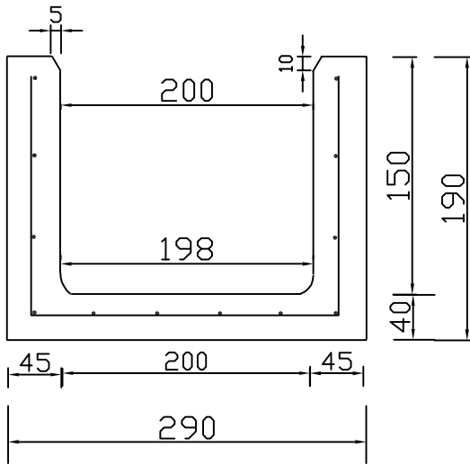
線槽側面及鋼筋透視圖
