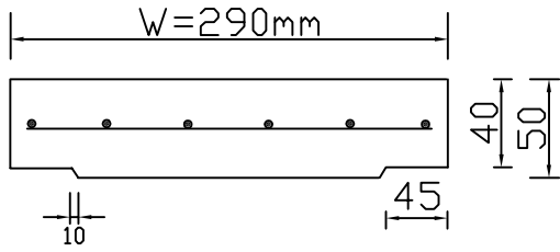
蓋板側面及鋼筋透視圖
