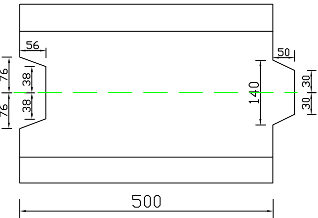
洋灰直型線槽俯視圖
