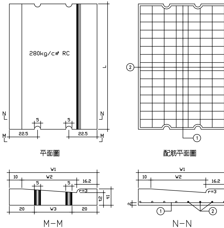
S 1 型預鑄溝蓋版各部尺寸及鋼筋表
