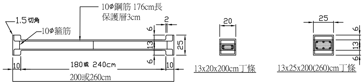
丁條詳圖
