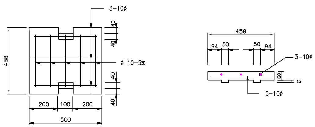
預鑄電纜槽蓋板 500×458×60mm
