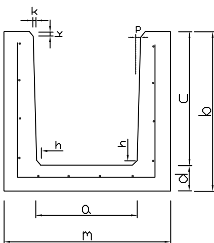
線槽側面及鋼筋透視圖
