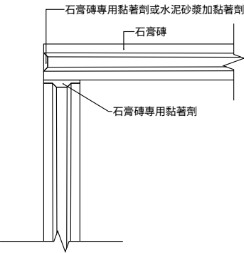
圖八 石膏磚 L型轉角剖面圖
