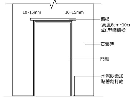
圖十一 石膏磚 門框上方楣樑施作圖
