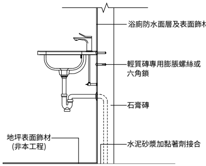
圖十八 石膏磚 浴室器具吊掛
