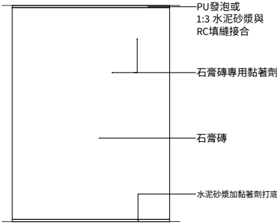
圖二 石膏磚 牆立面圖
