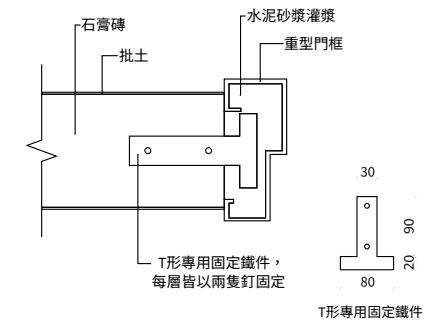
圖十四 石膏磚 門框先立固定圖 單位: mm
