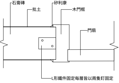
圖十三 石膏磚 與木門框固定圖二
