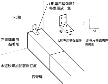
圖四 石膏磚 與 RC牆接和圖
