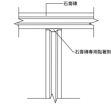
圖十 石膏磚 T型轉角剖面圖
