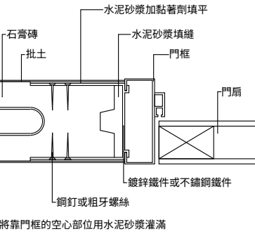
圖十五 石膏磚 門框後立固定圖 (工法一)
