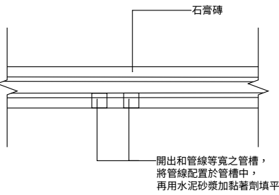
圖十七 石膏磚 水電管線配置
