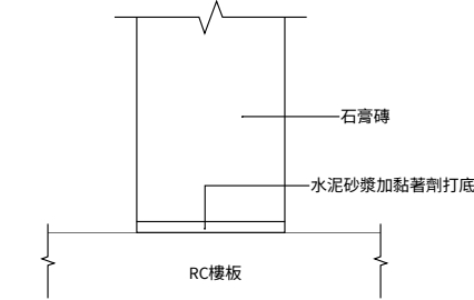
圖六 石膏磚 與 RC樓板接和剖面圖
