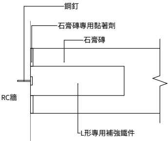
圖五 石膏磚 與 RC牆接和上剖面圖
