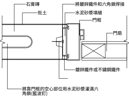
圖十六 石膏磚 門框後立固定圖 (工法二)
