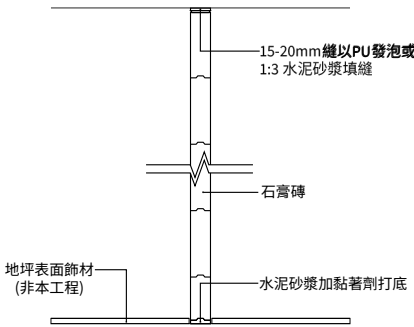
圖三 石膏磚 牆側面圖
