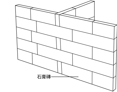
圖九 石膏磚 T型轉角立面圖
