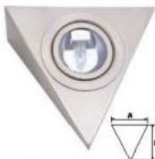
12V 20W (圓形變壓器) A:128mm B:143mm
