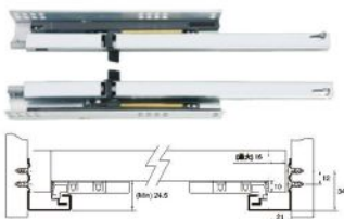
HM708 自動回歸緩衝三節抽底滑軌 (擺鉸式結合體)
