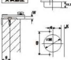
安裝底座
