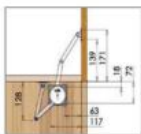
I3052 SUSPA 櫃體安全緩衝撐桿
