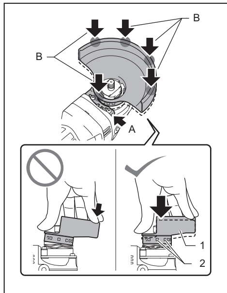
► 1. 砂輪罩 2. 開孔
