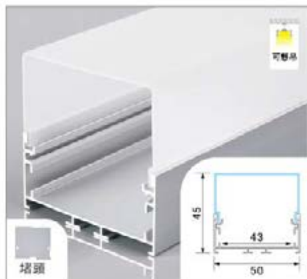
S5045三面發光
