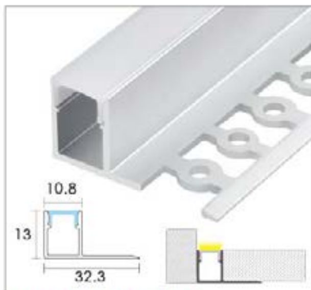
LD-H067 花邊預埋燈
