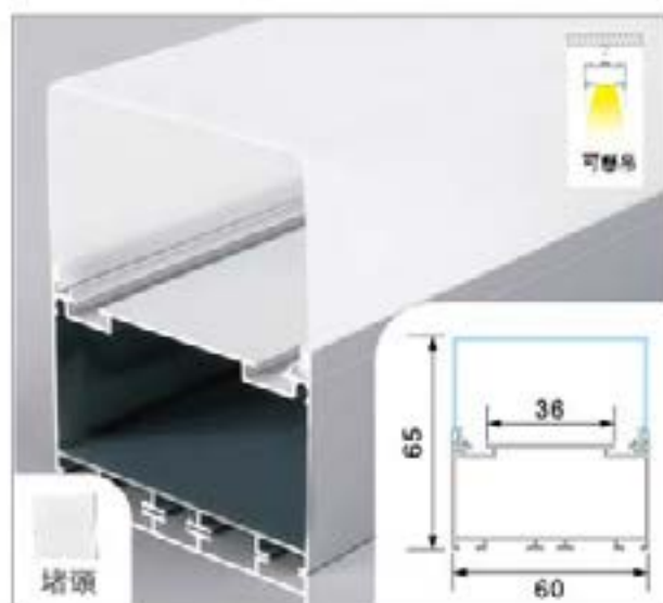
S6065三面發光
