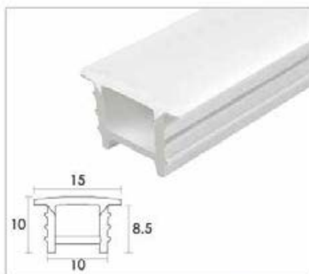
1010免穿燈帶矽膠 - 透明邊
