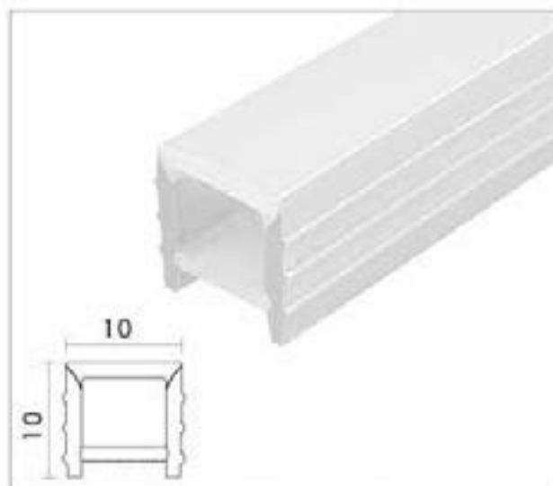
1010免穿燈帶矽膠 - 無邊
