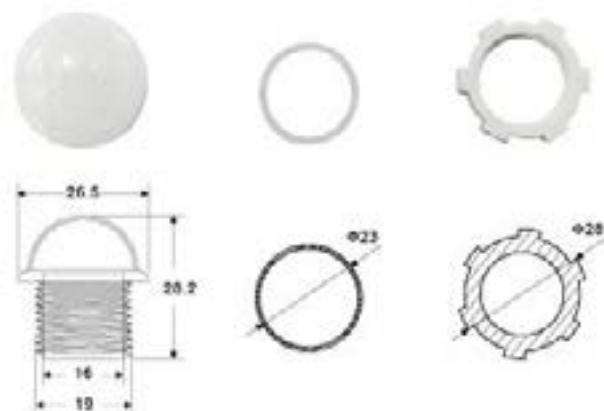
開關外觀尺寸圖：
