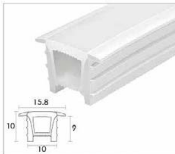
1010免穿燈帶矽膠 - 白邊
