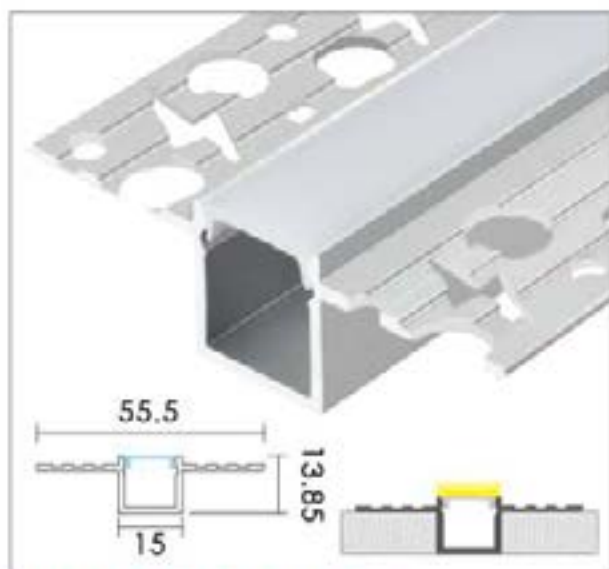
LD-H071 花邊預埋燈
