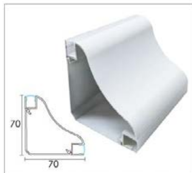
LD-H178 直角波浪形牆角燈
