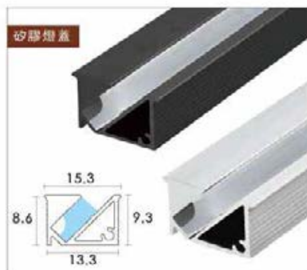
LAD1081 矽膠嵌入斜照燈
