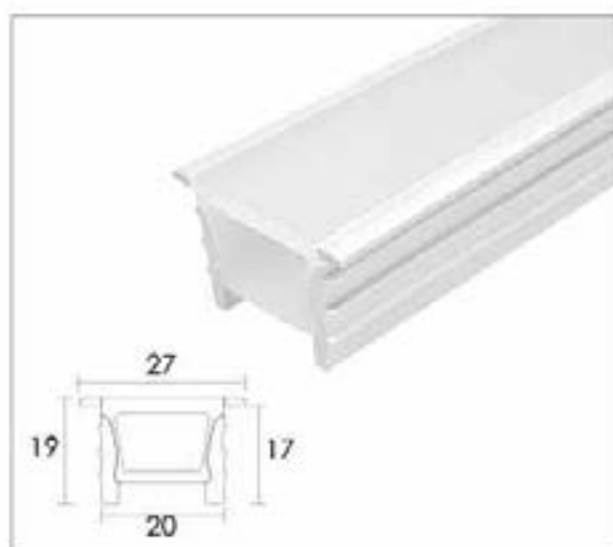
2020免穿燈帶矽膠 - 白邊
