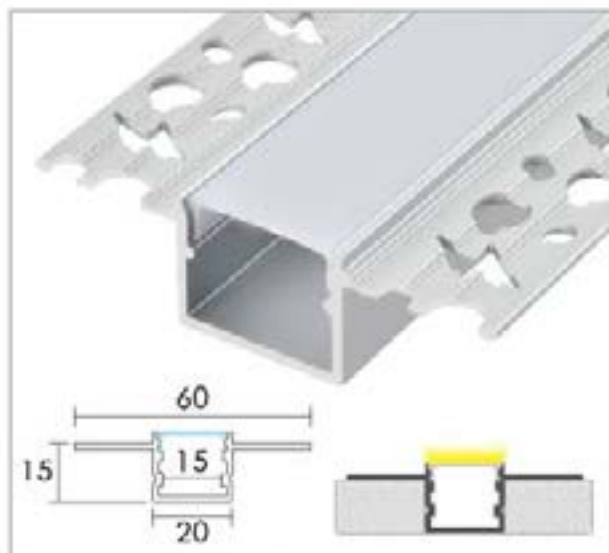
LD-H073 花邊預埋燈
