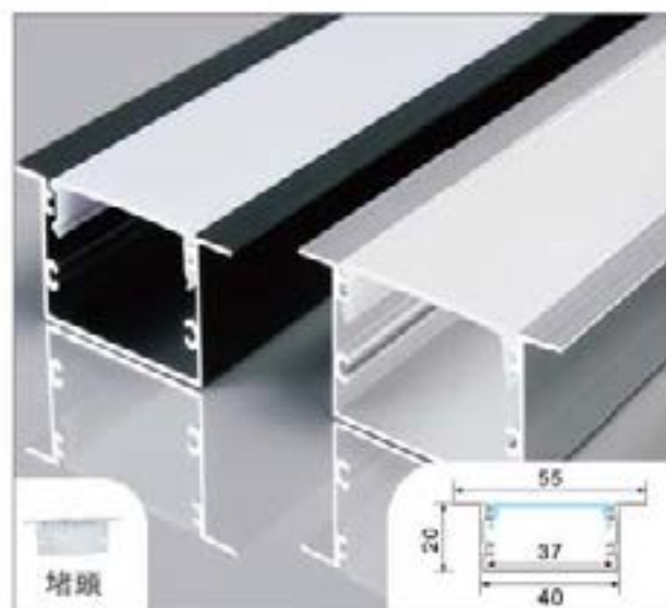
4020A單面發光
