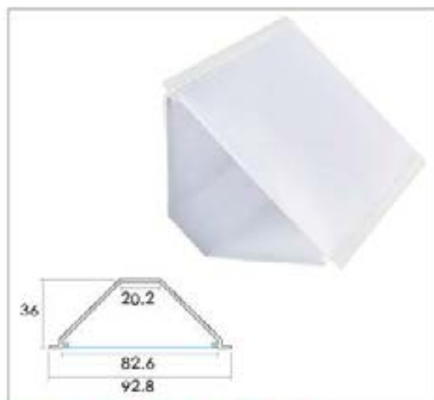
LD-Z608 主照明斜角燈
