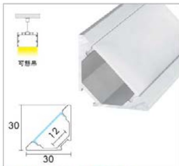
LD-S117 主照明斜角燈
