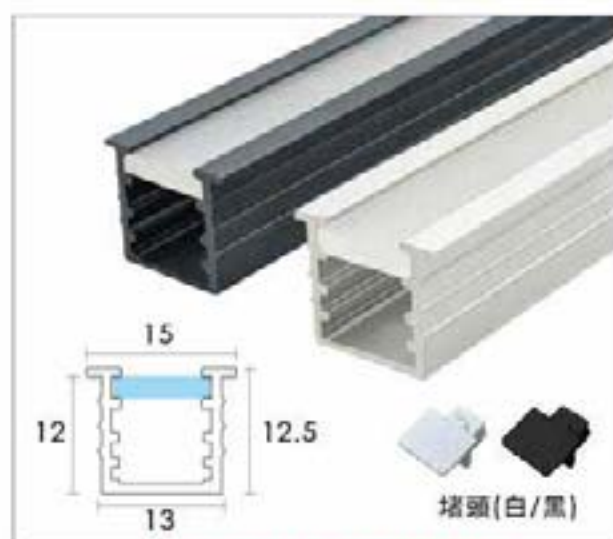
LAD0064 勻光嵌入硬條燈
