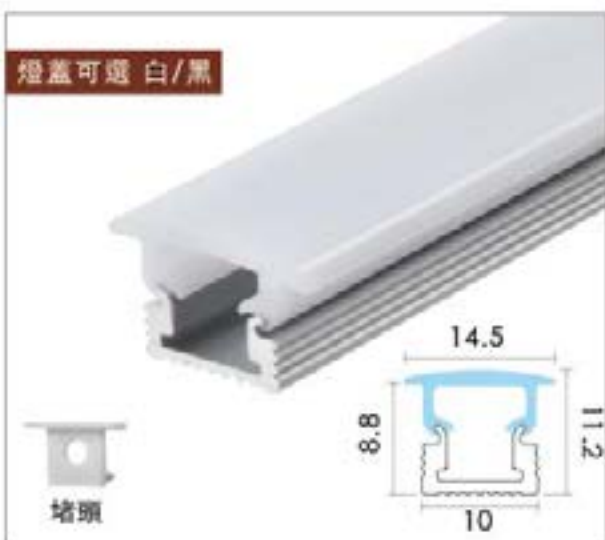
LAD0061 無邊嵌入硬條燈
