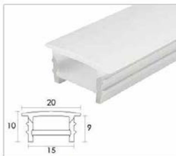
1510免穿燈帶矽膠 - 透明邊
