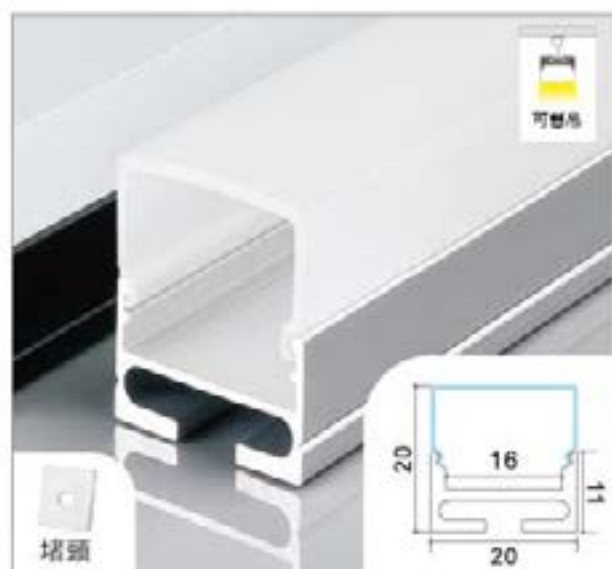
S2020三面發光
