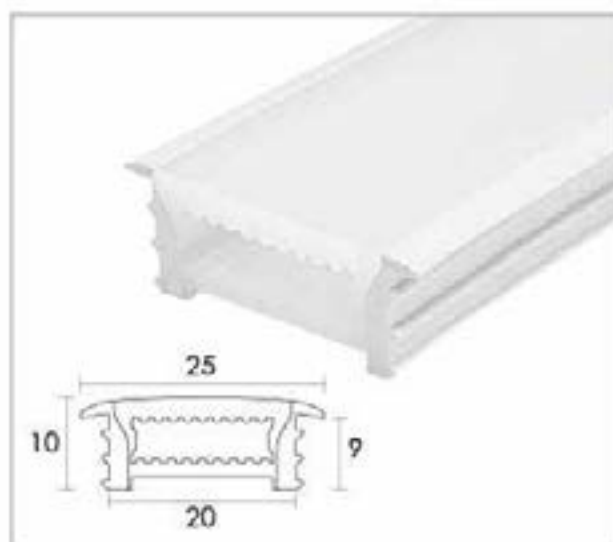
2010免穿燈帶矽膠 - 白邊
