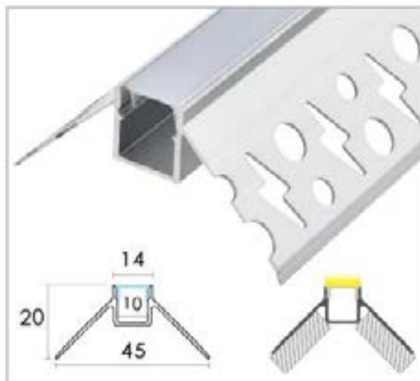
LD-H075 花邊預埋燈
