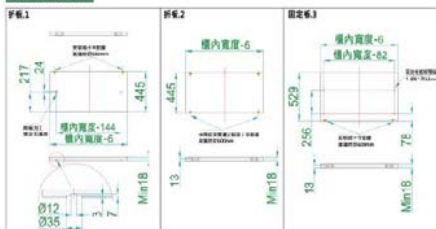
桌板操作參考尺寸:
