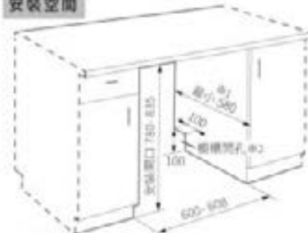
安裝空間
