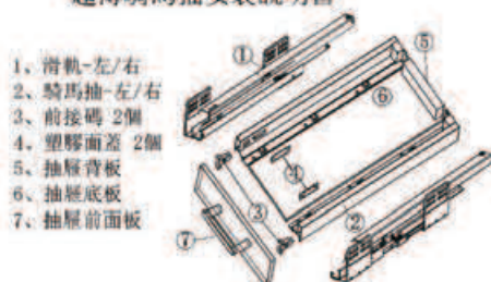
超薄騎馬抽安裝說明書
