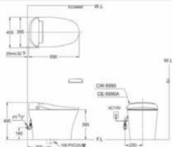
尺寸圖
