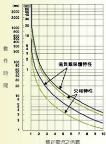
TH-P09PPS動作曲線特性
