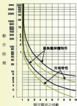
TH-P60(TA)/PP 動作特性曲線
