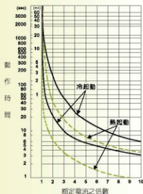
TH-P800N(E) 動作特性曲線
