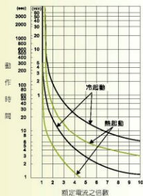
TH-P20(E)-6.5A以下 動作特性曲線
