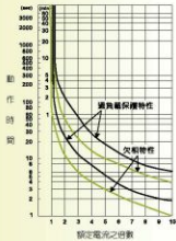
TH-P220(TP) - TH-P400(TP) 動作特性曲線
