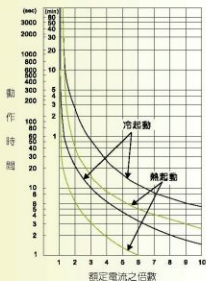
TH-P12(E) 動作特性曲線
