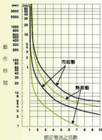
TH-P18(E)-9A以上 動作特性曲線
