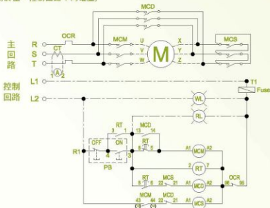
2.接線圖 (適用於主、控制回路不同電壓)
