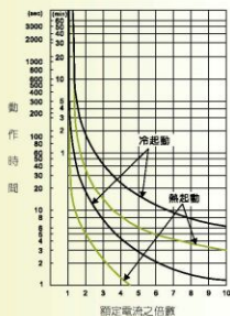
TH-P220T(E)・TH-P400T(E) 130A以下 動作特性曲線
