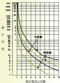
TH-P120(E)(TA) 動作特性曲線
