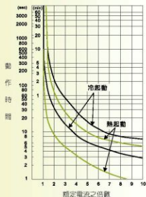
TH-P220T(E)、TH-P400T(E) 160A以上 動作特性曲線
