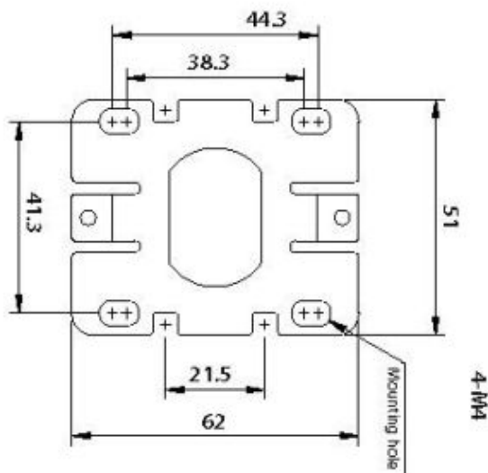
安裝尺寸(mm)
