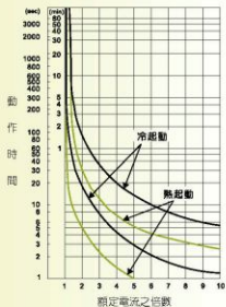
TH-P18(E)-6.5A以下 動作特性曲線
