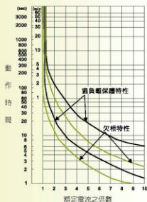
TH-P12PP 動作特性曲線
