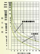
TH-P20(TA)/PP 動作特性曲線
