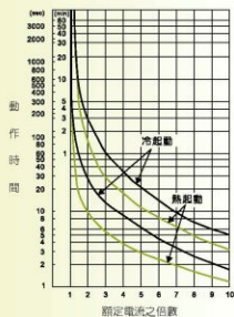
TH-P60(E)(TA) 動作特性曲線
