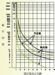
TH-P20(E)(TA)9A以上 動作特性曲線
