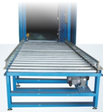
▲ 樓層式棧板輸送機
