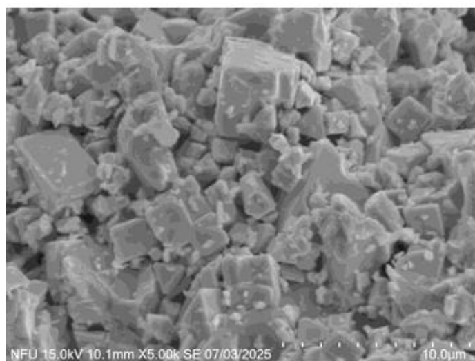
ZJ3017 的碳化鎢顆粒形貌
