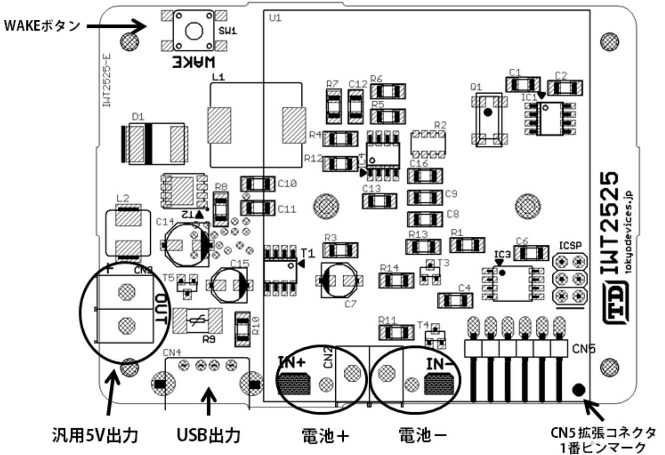
図 1 基板構成
