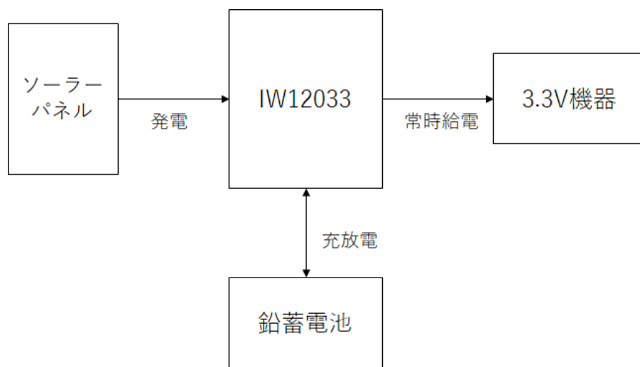
図 1 標準接続図
