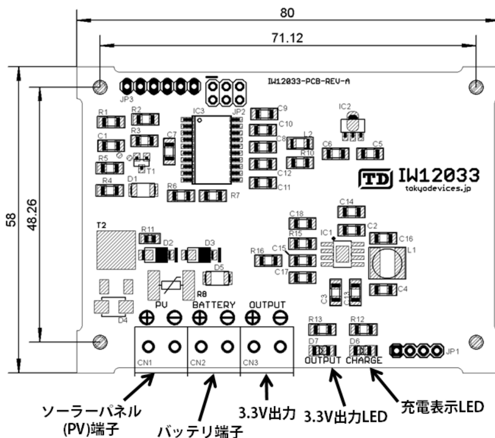
図 2 基板構成図
