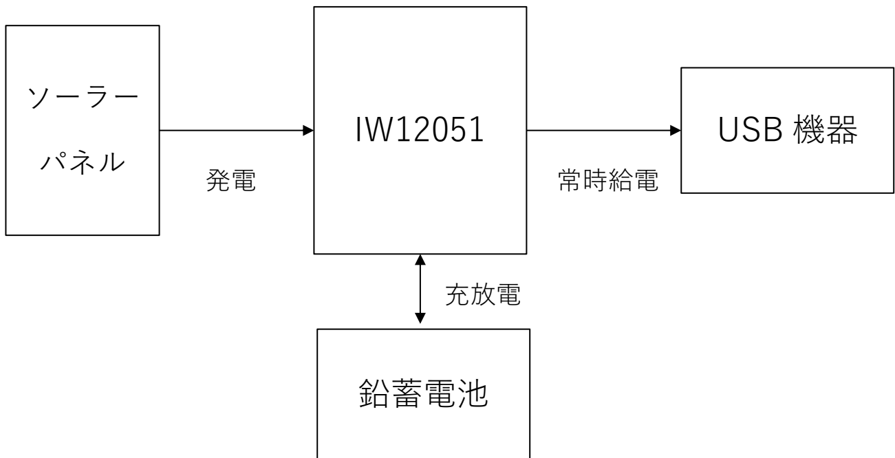
図 1 標準接続図
